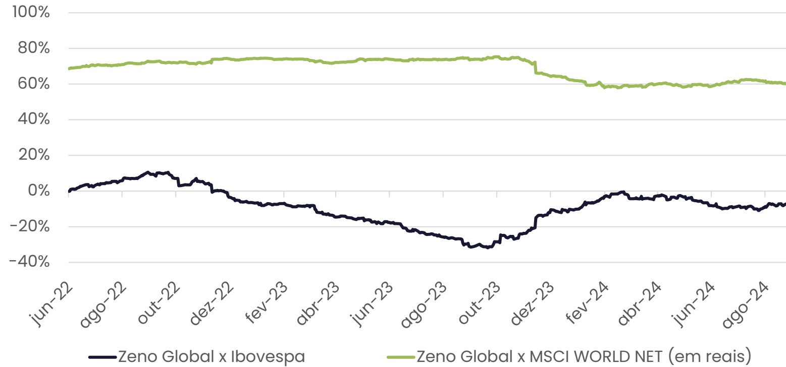
Retorno Acumulado (%)
