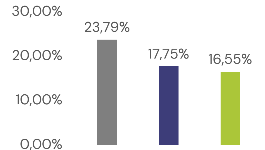
Vol Anualizada (%)
