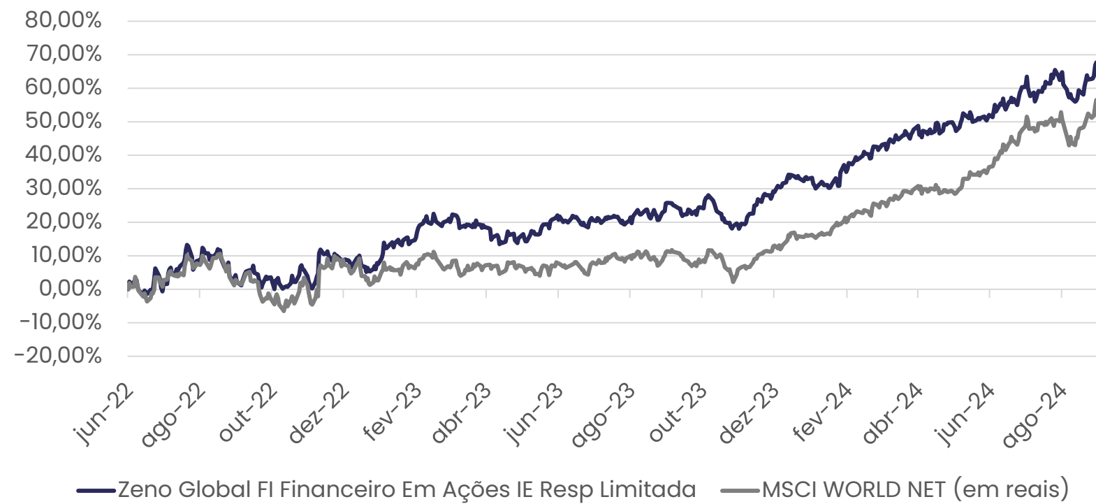
Retorno Acumulado (%)
