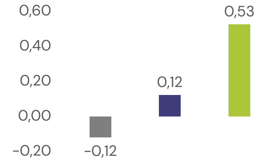
Vol Anualizada (%)
